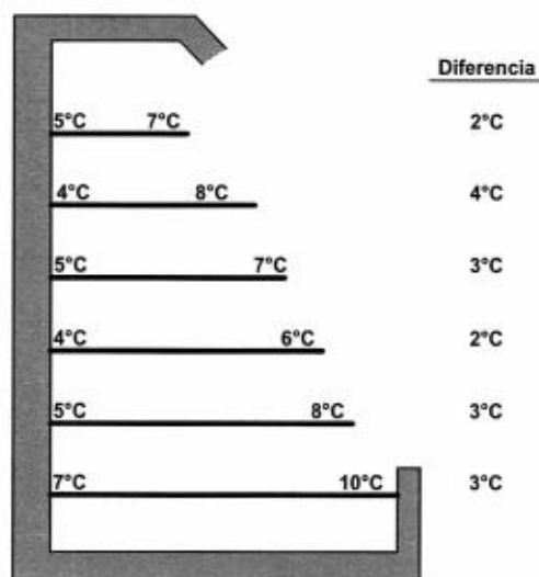
Figura 1. Diferencias de temperatura en estanterías abiertas típicas de supermercado. Fuente: Torres, 1989.
