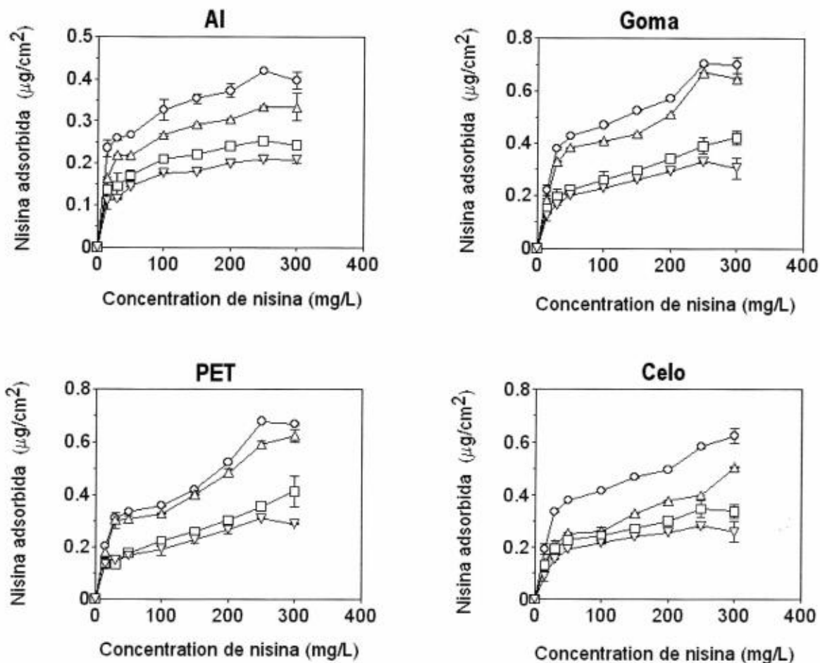
Figura 30: Isothermas de adsorción de la nisina a 8°C (○), 25°C (△), 40°C (□) y 60°C (▽) en superficies comúnmente usadas en la industria alimentaria: acero inoxidable (AI), goma, polietilentereftalato (PET) y celophane (Celo). Se han representado la media de los puntos experimentales (símbolos) con sus correspondientes desviaciones estándar (barras).
