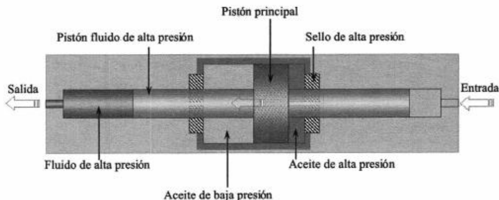
Figura 1. Tecnología de la bomba de alta presión (adaptada de Torres y Velásquez, 2004).
