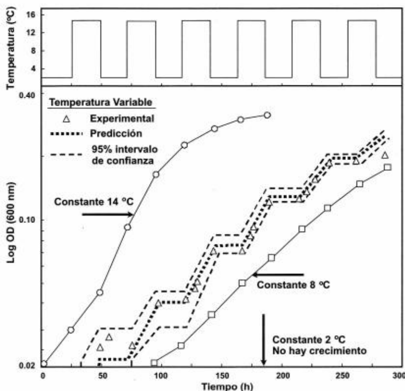
Figura 4. Predicción y determinación experimental de crecimiento microbiano bajo fluctuaciones de temperatura ( Brochothrix thermosphacta en medio líquido de cultivo).
