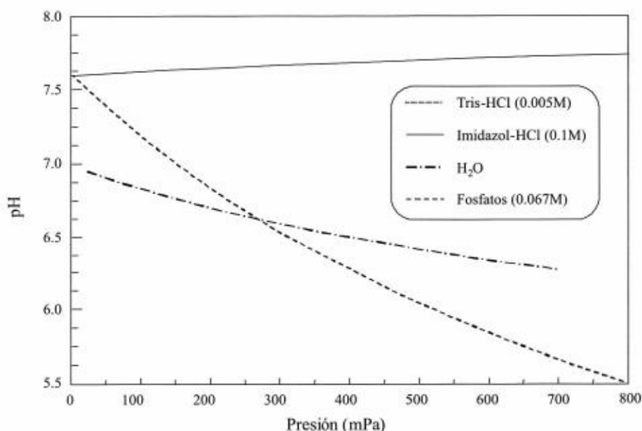
Figura 6. Cambios en el pH del medio inducidos por la presión ( http://www.tu-berlin.de/fb15/institute/lmt1/dahlem/html/body_high_pressure.html )
