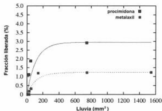
Figura 7. Datos observados (símbolos) y modelo de liberación de primer orden (líneas) para el metalaxil y la procimidona; fracción liberada frente a lluvia acumulativa.
